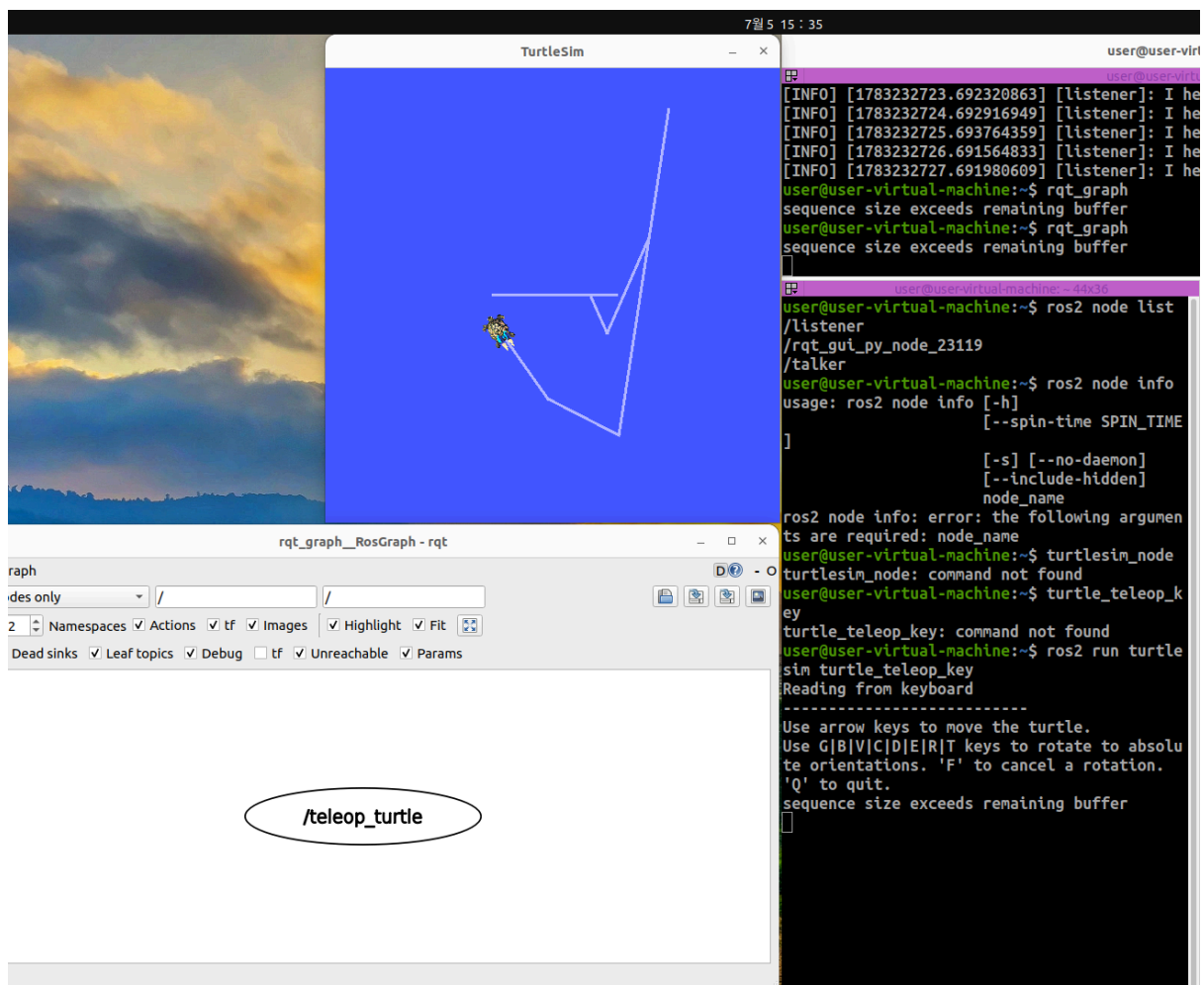
그림2) 터틀심을 움직이는 노드
